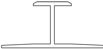
Actual
